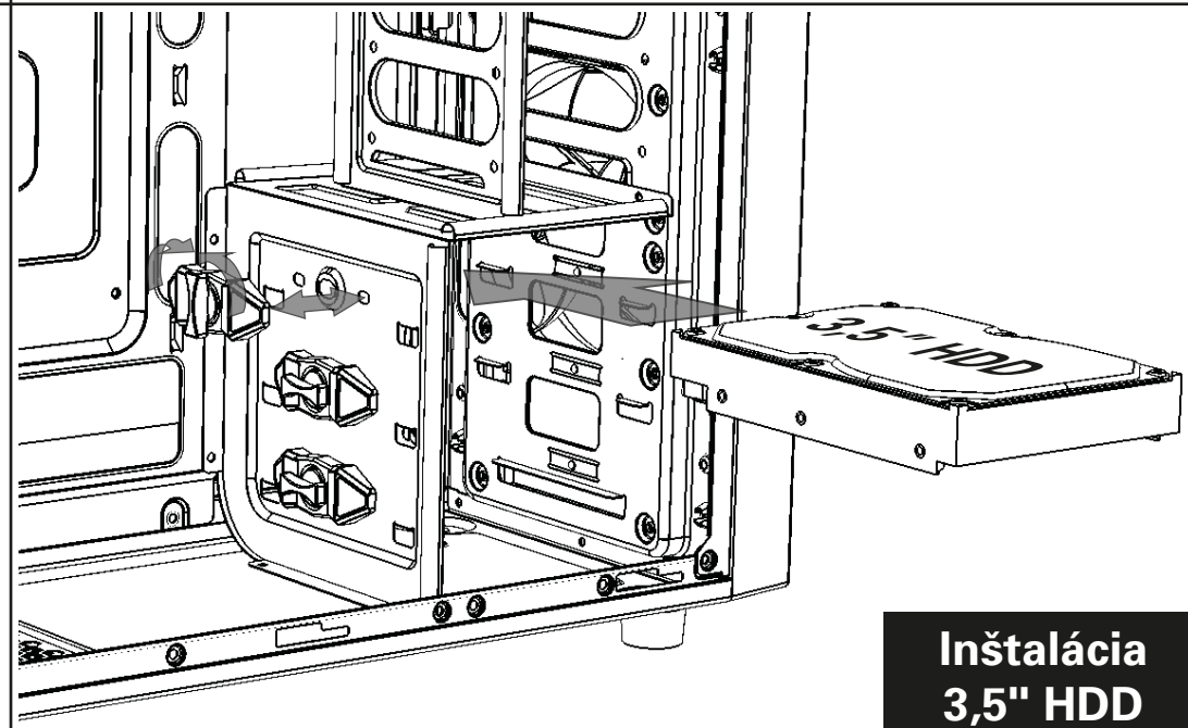
Inštalácia 3,5" zariadenia
